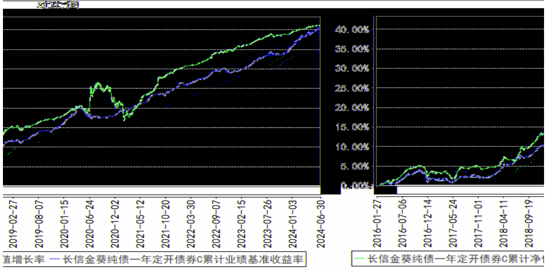
长信金葵纯债一年定开债券C累计净值增长率与同期业绩比较基准收益率的区间走势图
